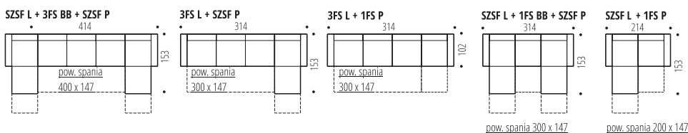
Schemat rozkładania funkcji spania typ. DL www.mpnidzica.pl
